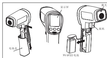
图 2. 红外测温仪
